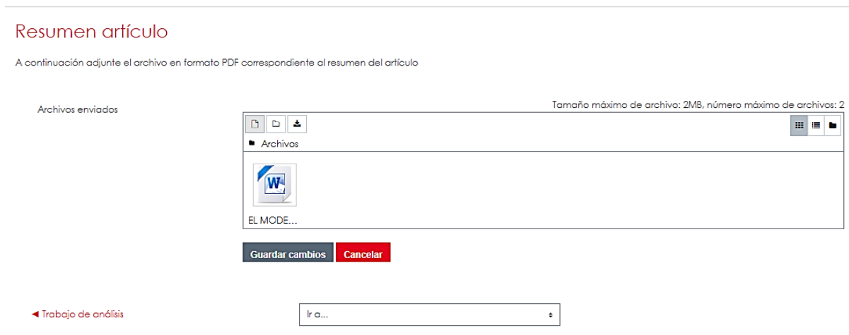
Figura 22. Guardar cambios
